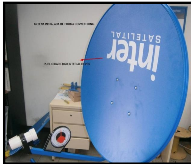
Imagen 26. Ensamble convencional de la antena invertida
