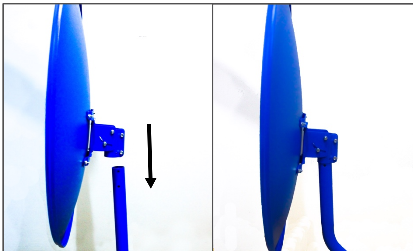
Imagen 19. Armado de Antena Inter Satelital.
